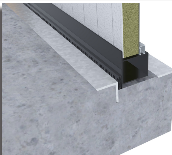
Detail onderdorpel BGS en AV deuren
