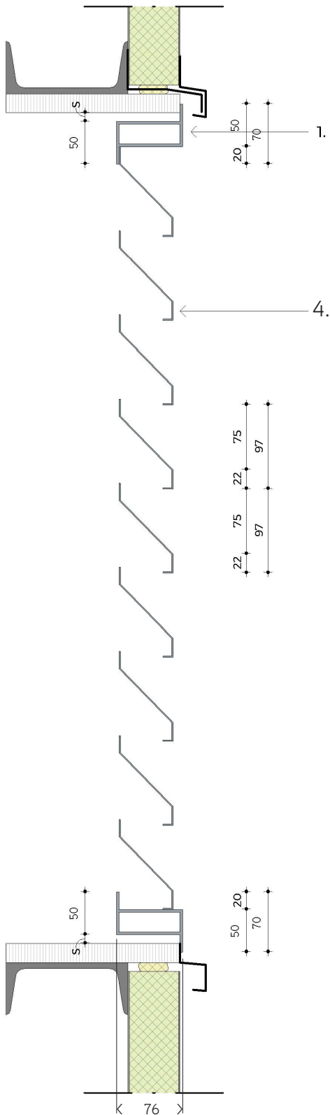
Lamellenrooster
